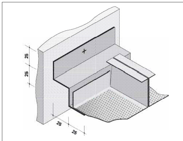
Shadow edge trim 25 x 25 x 25 x 1.0 mm steel
